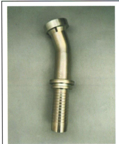
87933CAT 45° SAE FLANGE 9000PSI
