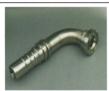
87693 90° SAE FLANGE 6000PSI Six layer
