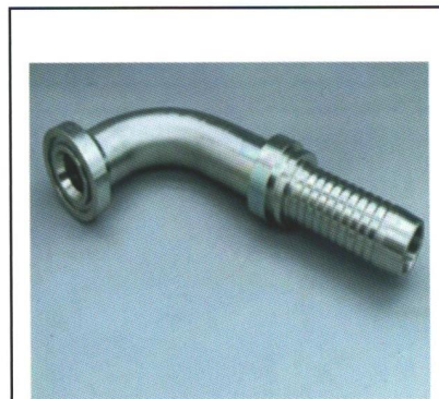
87692VOIVO 90° SAE FLANGE 6000PSI
