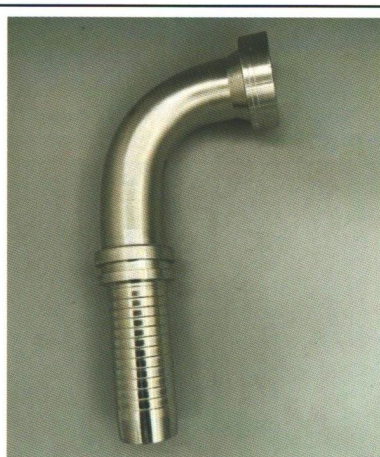
87993L 90° SAE FLANGE 9000PSI
