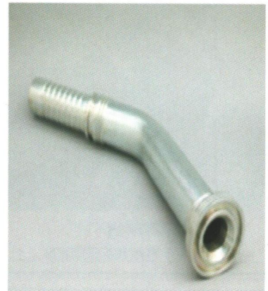
87342H 45° SAE FLANGE 3000PSI
