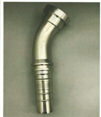
87943 45° SAE FLANGE 9000PSI Six layer
