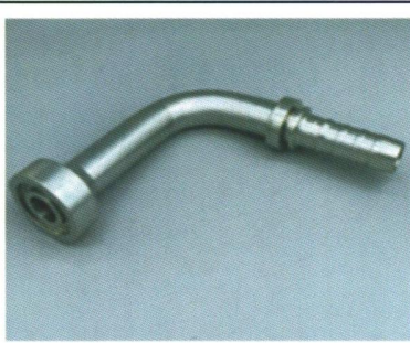
87992-16H130 SAE FLANGE 9000PSI (CAT)
