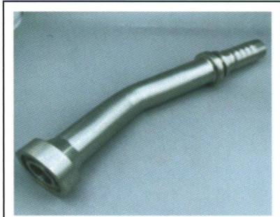
87932-16/12(H100=100) (16/12)30° SAE FLANGE 9000PSI (CAT)
